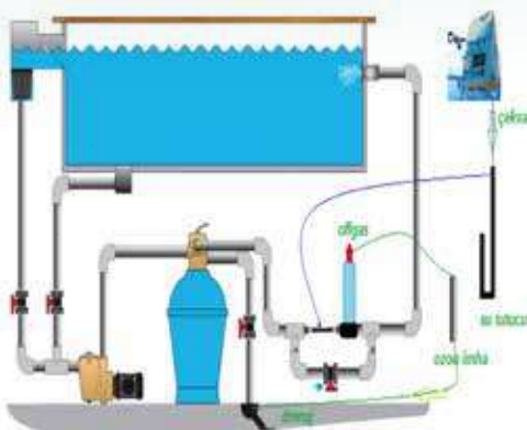
DOZON MINI DEGASTOR ASSEMBLY DIAGRAM
