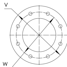
DISCHARGE FLANGE
